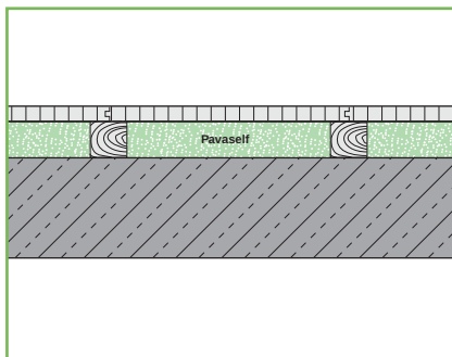
Vullen van holle ruimtes onder houten vloeren
