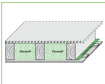
Isolatie tussen de balken
